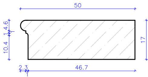
presjek
